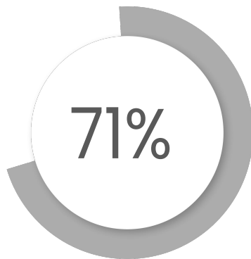
GitHub Copilot
