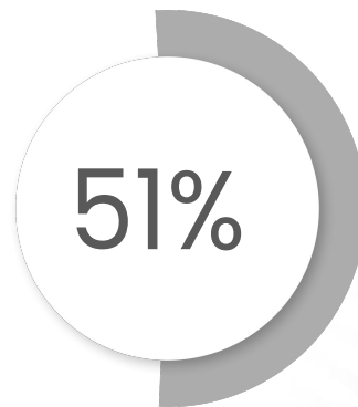
Cursor (Auto)
